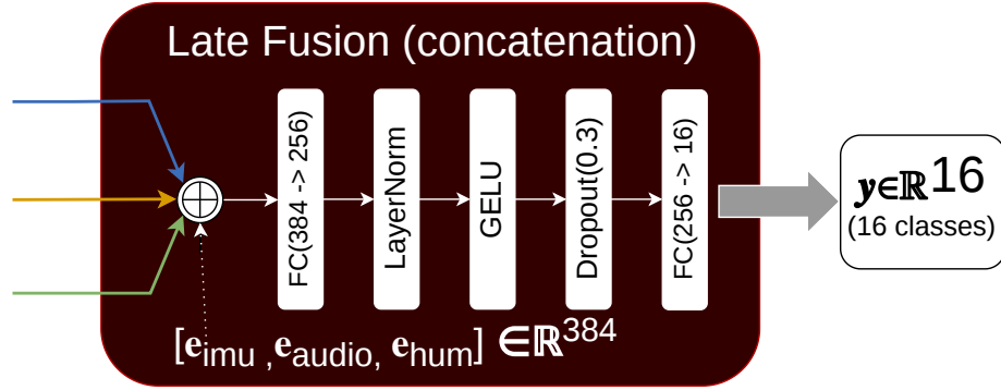
Fig. 10. Late Fusion (concatenation)
